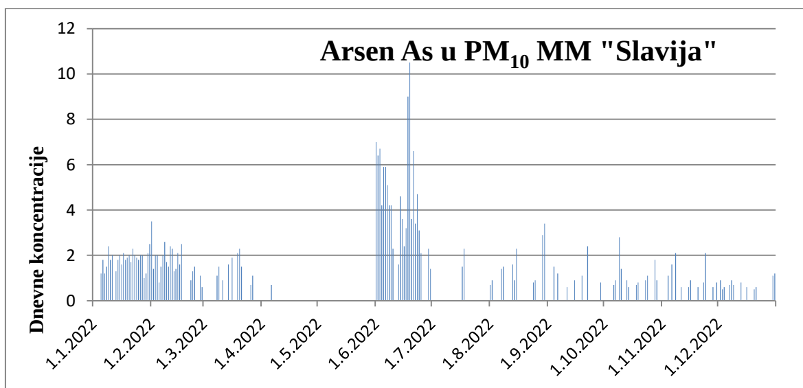
Grafik 5. Rezultati As u PM 10 , na MM „Slavija“ 2022.
