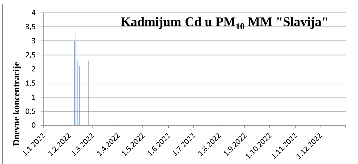
Grafik 5. Rezultati Cd u PM 10 , na MM „Slavija“ 2022.
