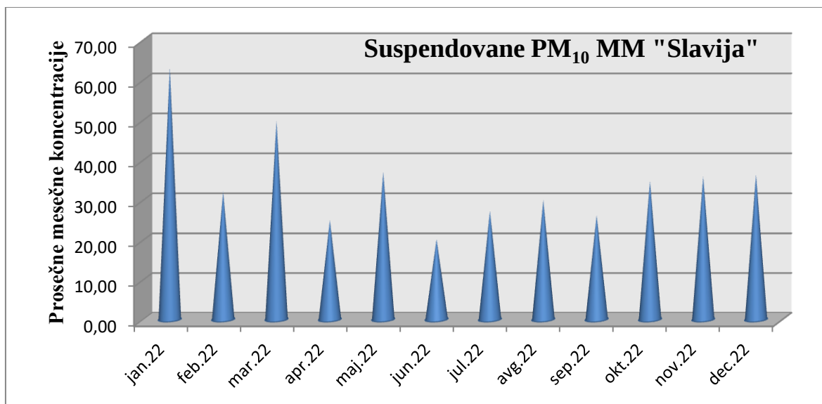
Grafik 2. Trend srednjih vrednosti suspendovanih materija PM 10 , na MM „Slavija“ 2022.
