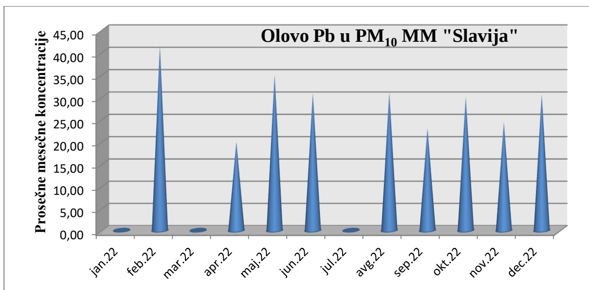
Grafik 4. Trend srednjih vrednosti Pb u PM 10 , na MM „Slavija“ 2022.
