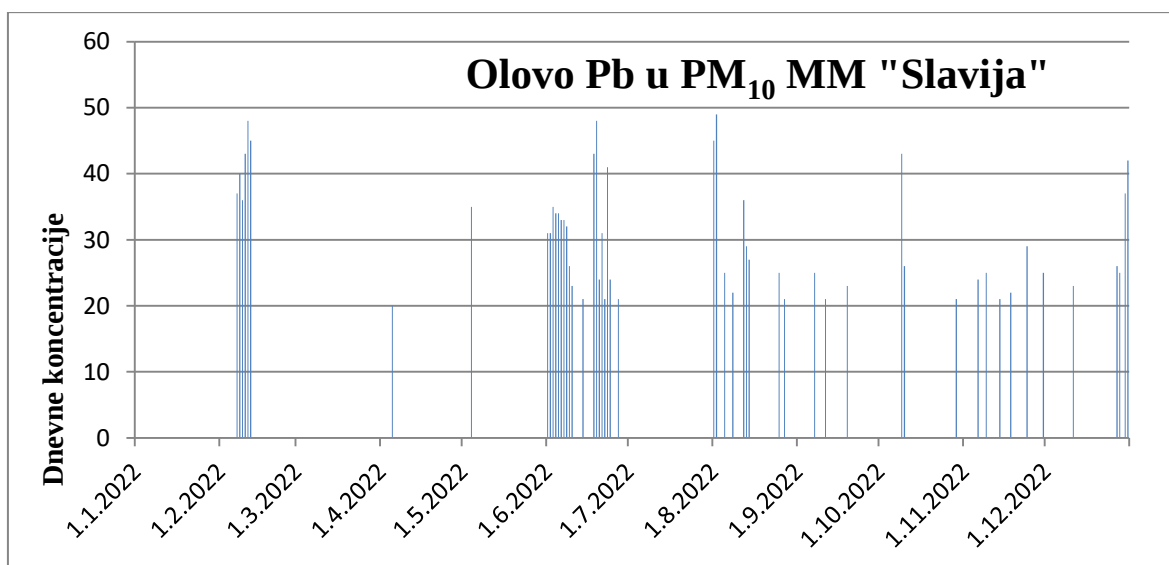
Grafik 3. Rezultati Pb u PM 10 , na MM „Slavija“ 2022.
