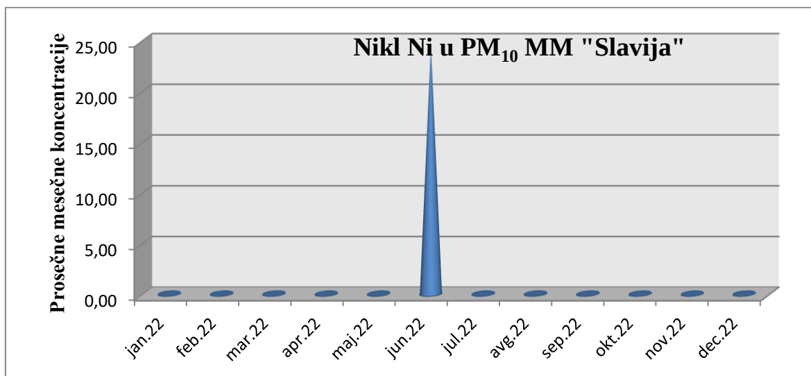
Grafik 8. Trend srednjih vrednosti Ni u PM 10 , na MM „Slavija“ 2022.
