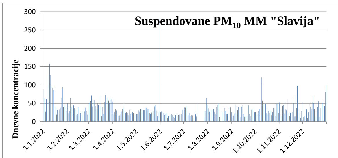
Grafik 1. Rezultati suspendovanih materija PM 10 , na MM „Slavija“ 2022.
