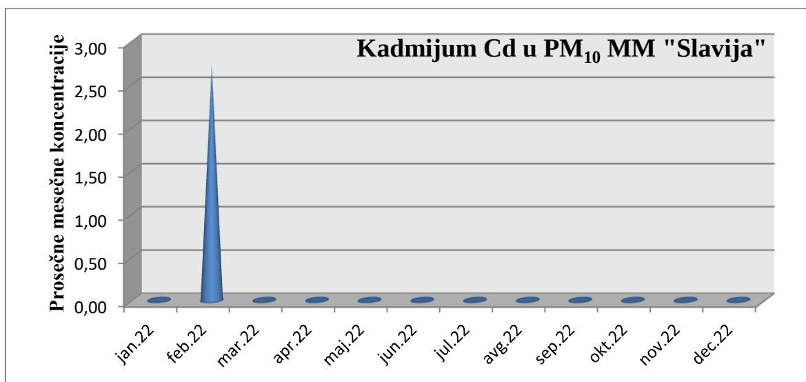
Grafik 6. Trend srednjih vrednosti Cd u PM 10 , na MM „Slavija“ 2022.
