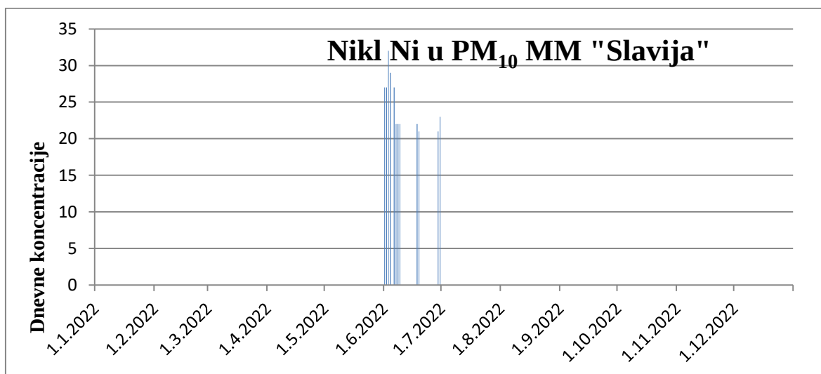
Grafik 7. Rezultati Ni u PM 10 , na MM „Slavija“ 2022.
