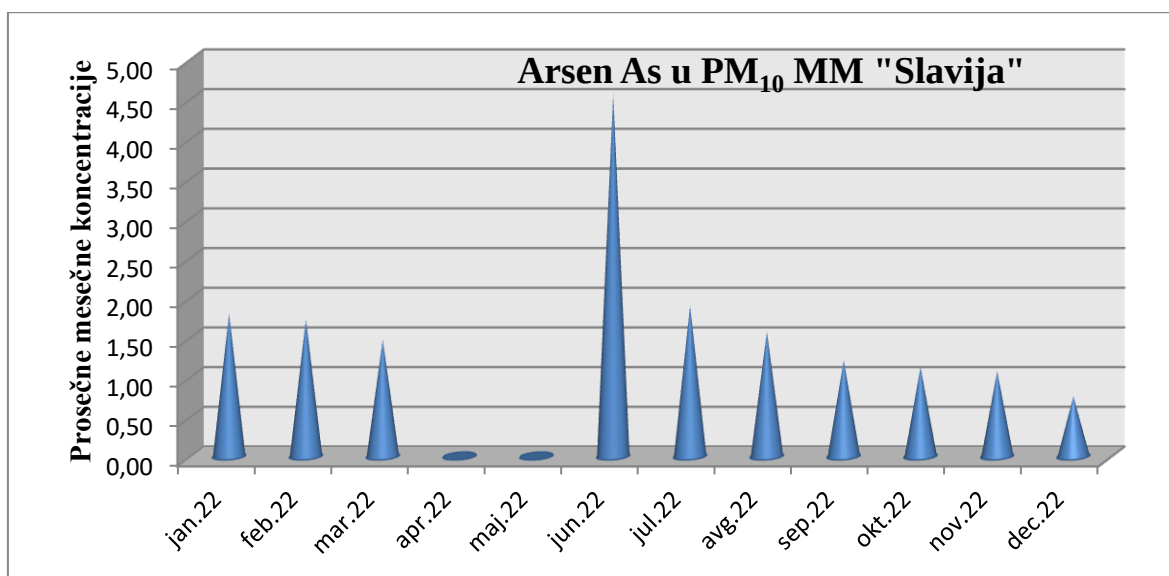
Grafik 6. Trend srednjih vrednosti As u PM 10 , na MM „Slavija“ 2022.
