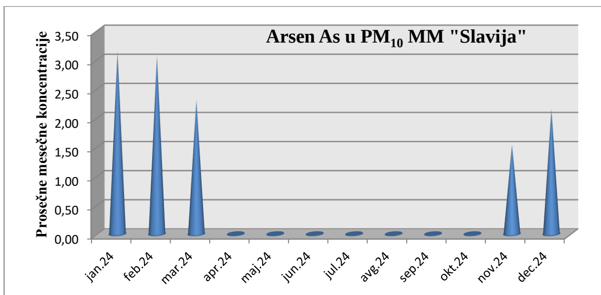
Grafik 6. Trend srednjih vrednosti As u PM 10 , na MM „Slavija“ 2024.
