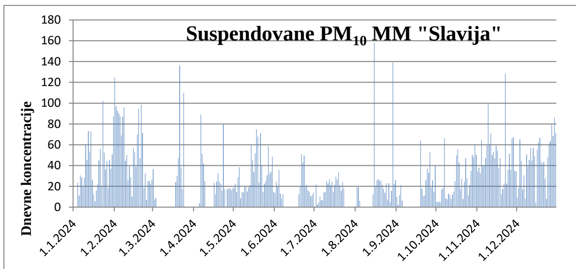
Grafik 1. Rezultati suspendovanih materija PM 10 , na MM „Slavija“ 2024.
