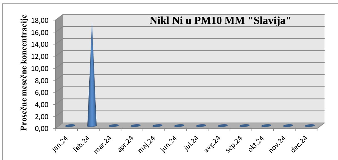
Grafik 8. Trend srednjih vrednosti Ni u PM 10 , na MM „Slavija“ 2024.
